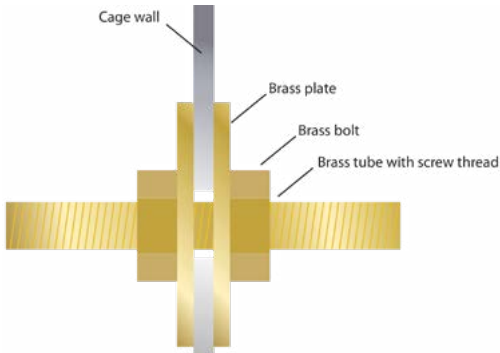
Waveguide brass 7855-11,62 & 7855-20,80
