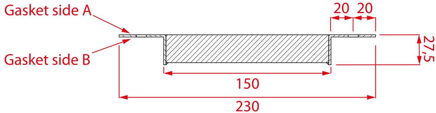
A-A ( 1 : 2 )
